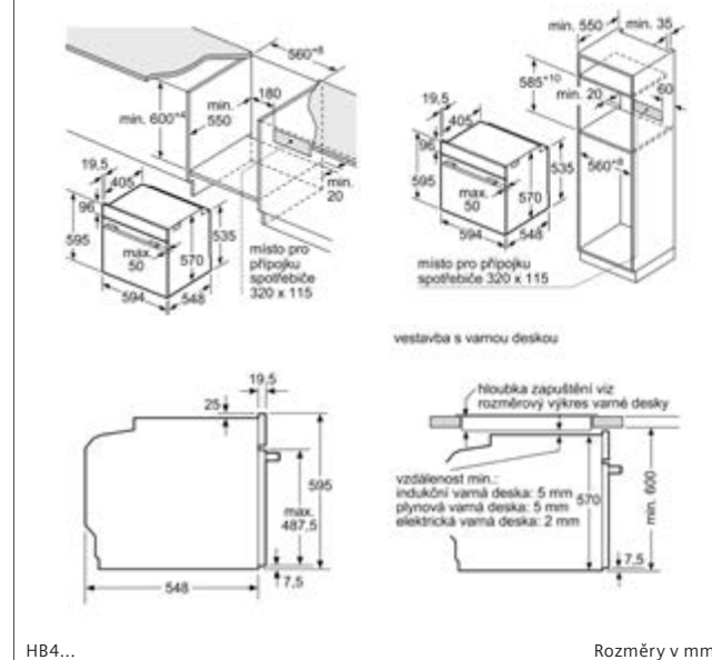
Pečící trouba
